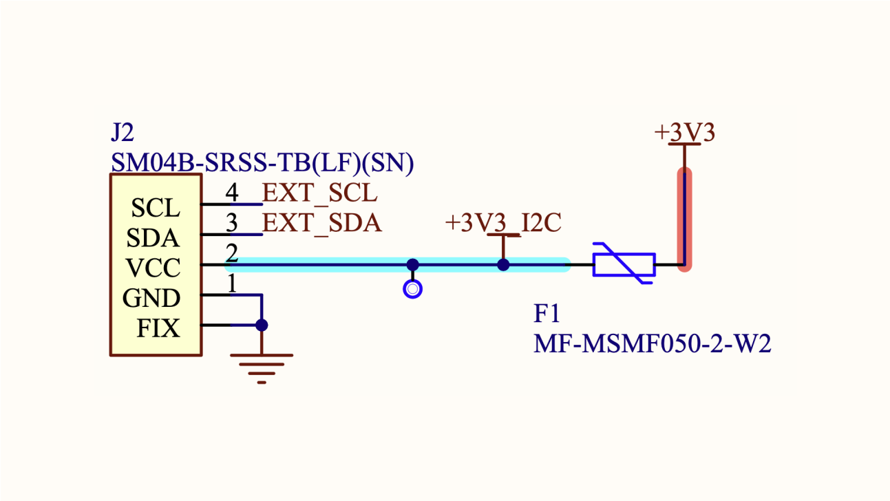
I2C模块。
